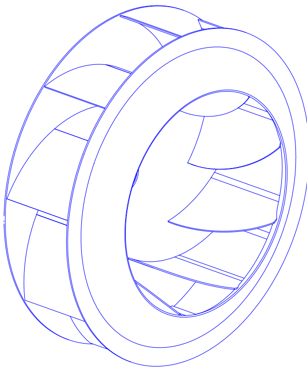
Колесо рабочее вентилятора ВР 80-75/9
